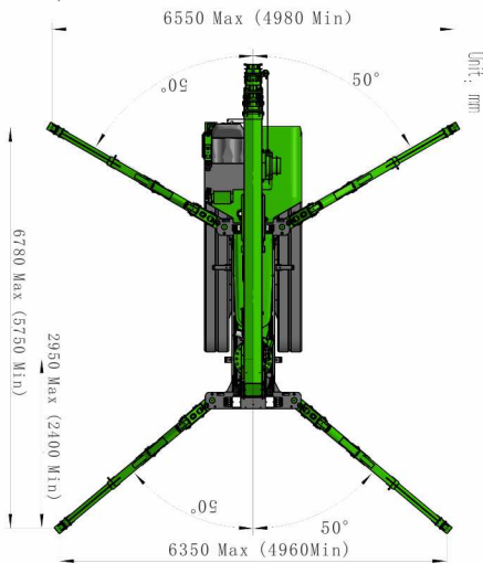
展开尺寸
