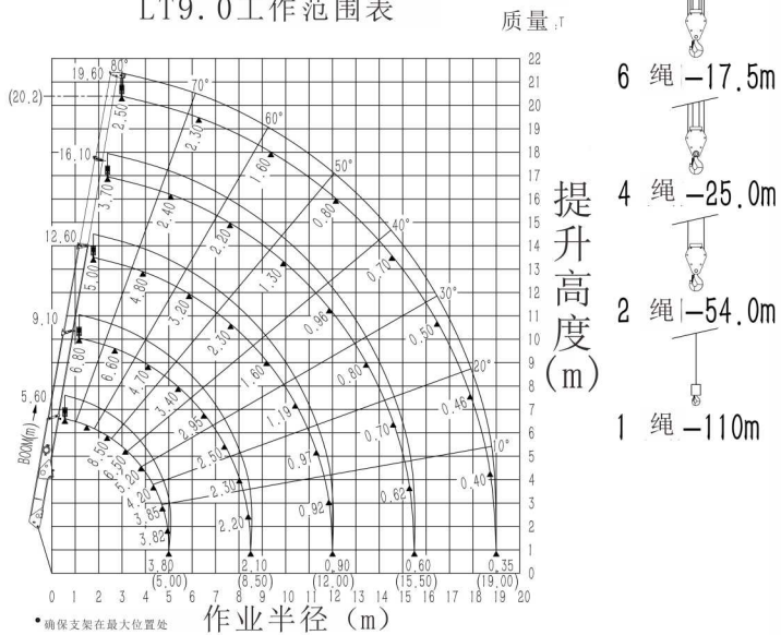
LT9.0工作范围表
